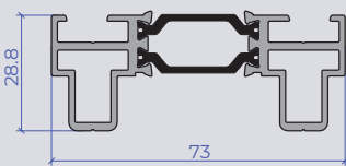
Adjustable jamb
