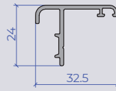
Swing door rebate
